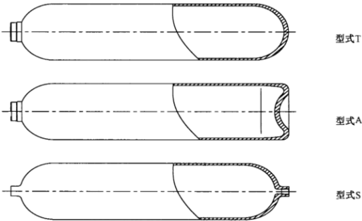
图 1 钢瓶瓶体结构型式
